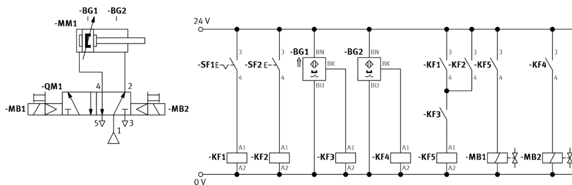
2 - Diagram pro elektro-pneumaticky ovládaný systém
